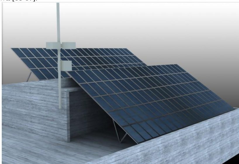
Slika 5. Idejno rešenje instalacije solarnih panela na krovu opštine Vračar
